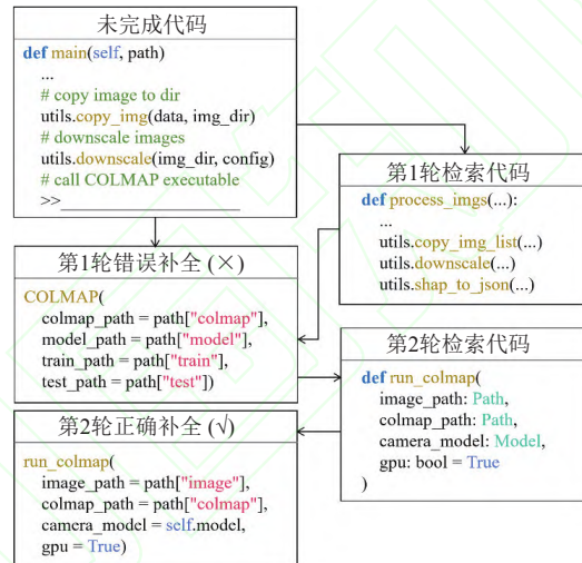
图6 迭代的检索-生成循环示例 [38]
