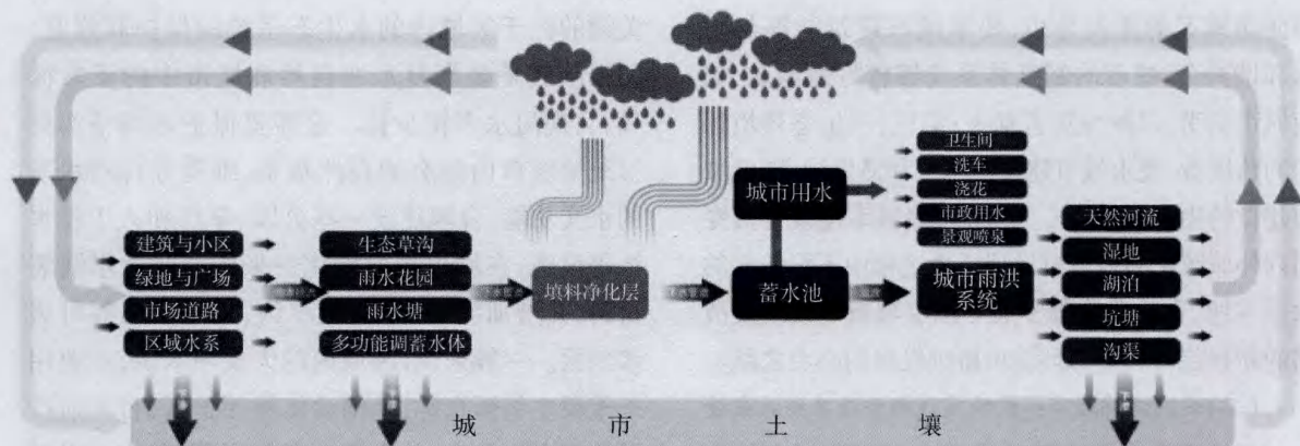
图5 海绵城市水循环流程图解
