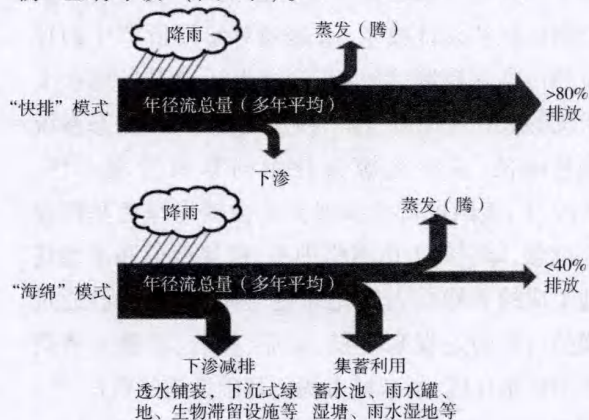
图1 传统快排模式与海绵排放模式
